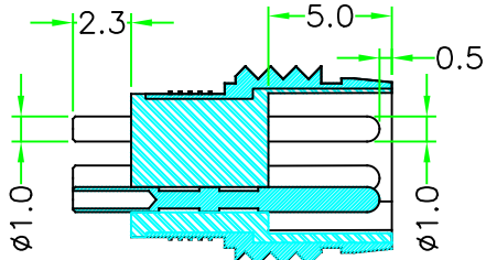
剖面圖 A-A
