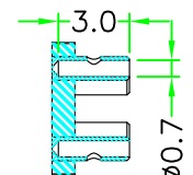
剖面圖 A-A
